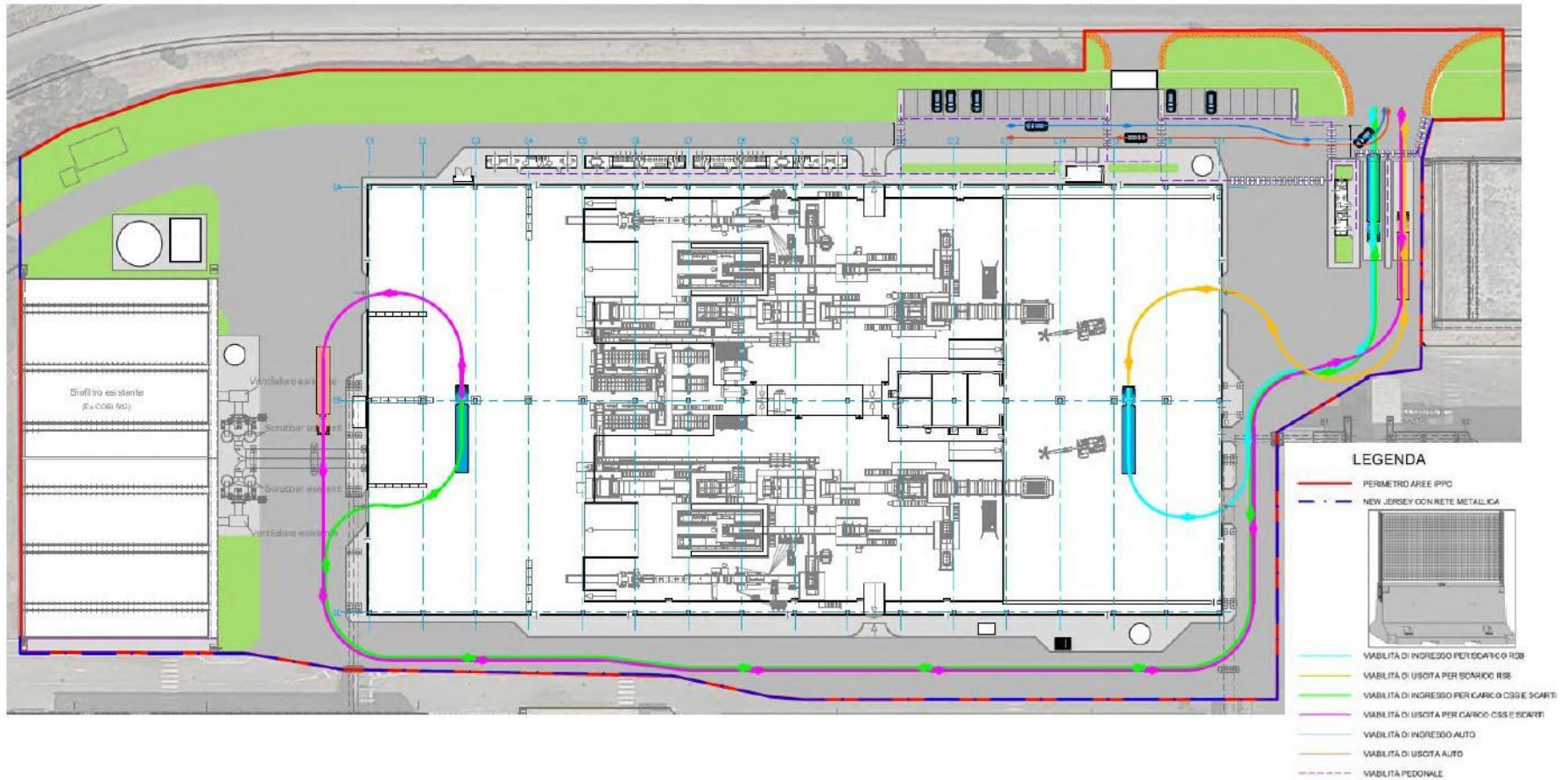
Figura 1: Planimetria dell'impianto con perimetro.
