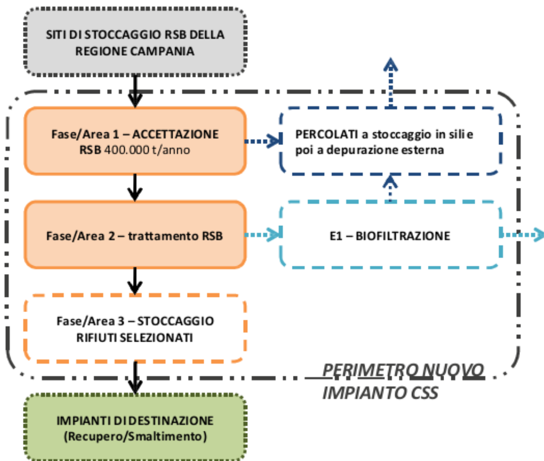
Figura n° 2–Schema a blocchi del processo
