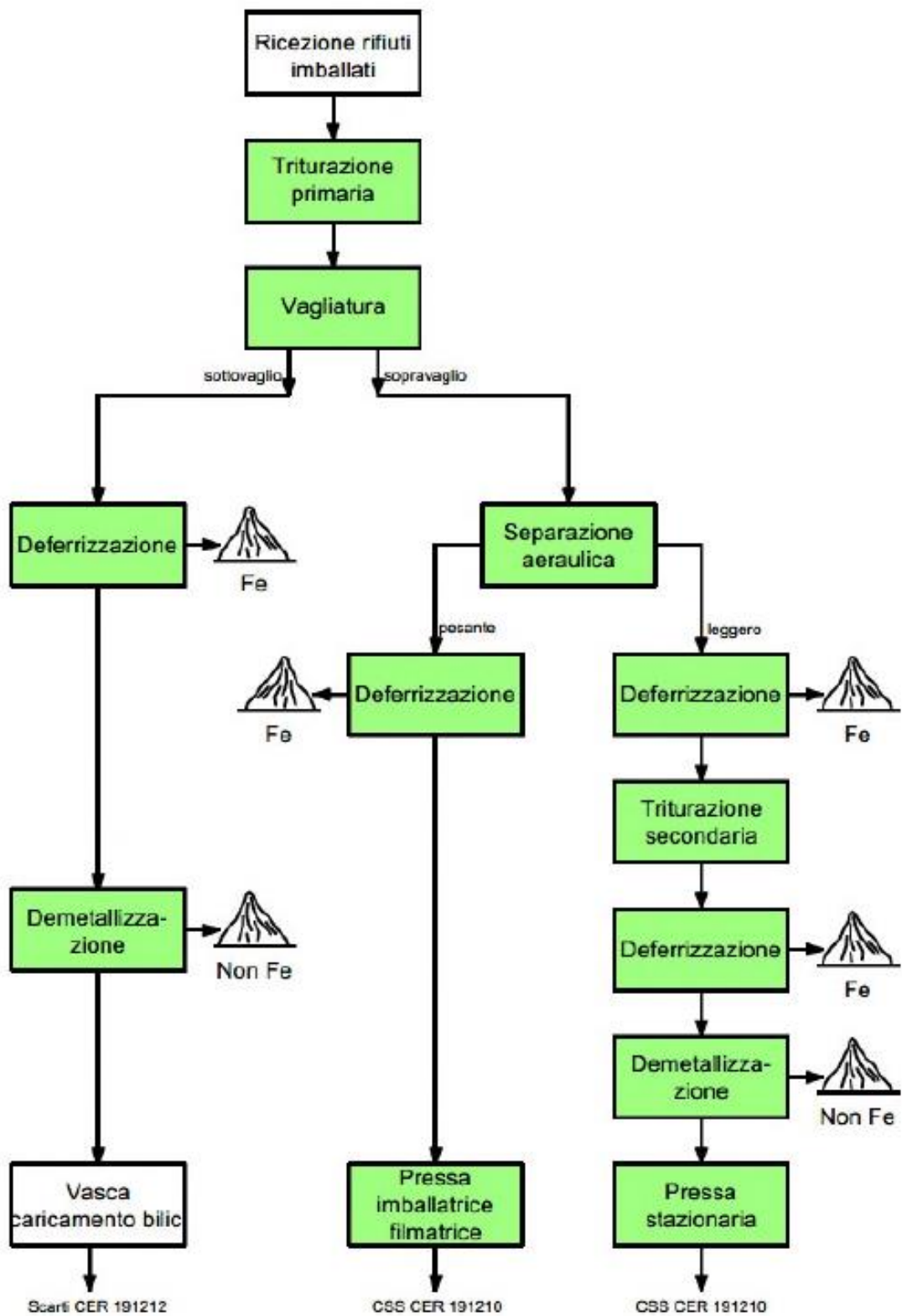
Figura n° 3–Schema a blocchi delle unità di trattamento
